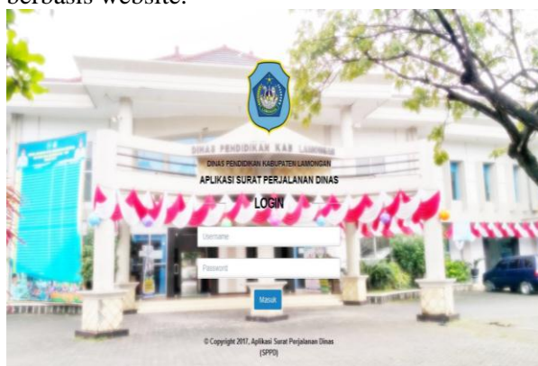
Gambar 8. Tampilan Login
