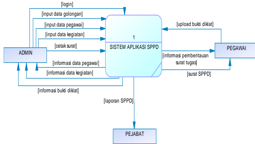
Gambar 1. Diagram Konteks
