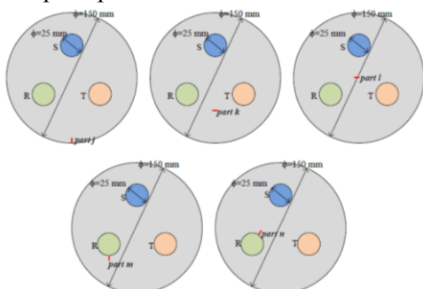
Gambar 6. Posisi partikel dalam model GIS 3 fasa susunan equilateral
