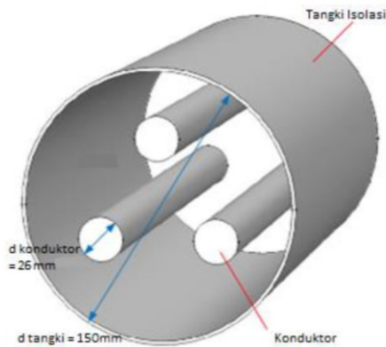
Gambar 3. Model busbar berisolasi gas SF6 pada GIS equilateral 3 fasa
