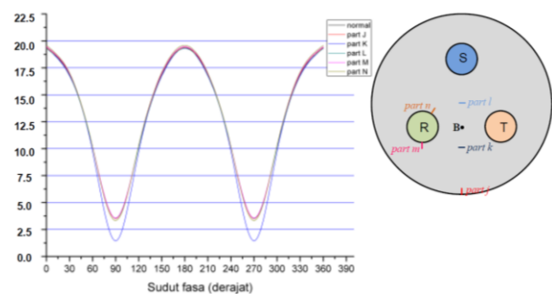
Gambar 15. Medan listrik di titik B dengan keberadaan partikel asing pada posisi yang berbeda-beda
