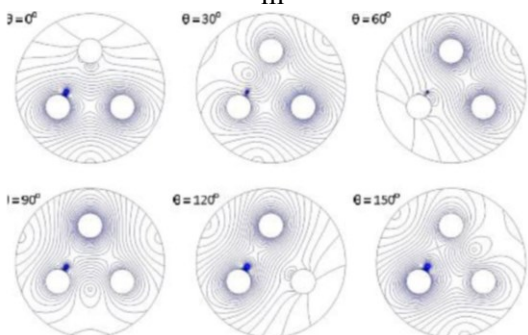
Gambar 12. Distribusi medan listrik dalam tangki GIS equilateral dengan keberadaan partikel n
