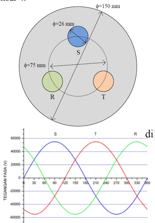
Gambar 4. Deskripsi model GIS tiga fasa yang disederhanakan dan tegangan masing-masing konduktor.
