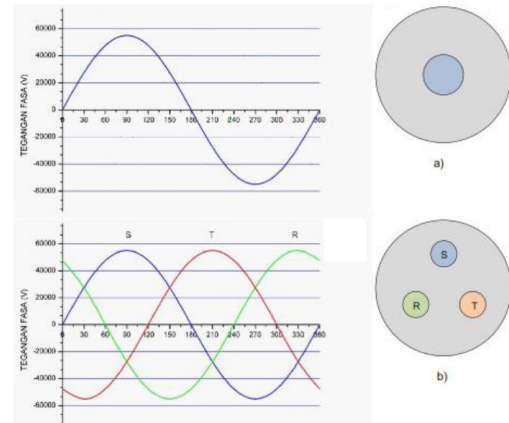
Gambar 2. Konfigurasi dan tegangan kerja peralatan satu fasa dan tiga fasa.
