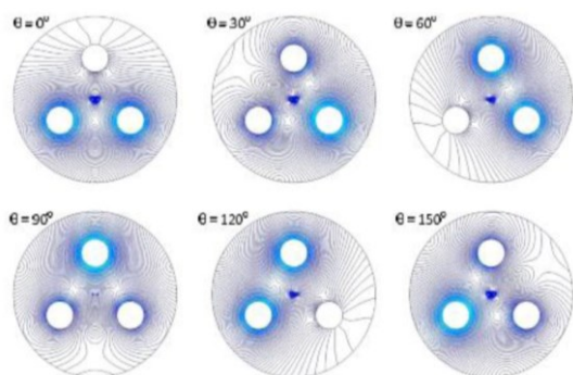
Gambar 10. Distribusi medan listrik dalam tangki GIS equilateral dengan keberadaan partikel l
