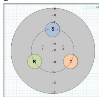
Gambar 5. Posisi titik tinjau medan listrik dalam model GIS 3 fasa susunan equilateral
