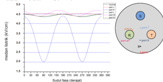
Gambar 17. Medan listrik di titik D dengan keberadaan partikel asing pada posisi yang berbeda-beda
