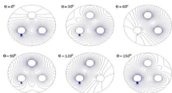
Gambar 11. Distribusi medan listrik dalam tangki GIS equilateral dengan keberadaan partikel m
