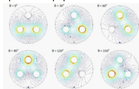
Gambar 7. Distribusi medan listrik dalam tangki GIS equilateral tanpa partikel
