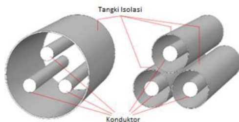
Gambar 1. Konstruksi GIS 3 Fasa dan GIS 1 Fasa
