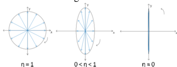
Gambar 20. Bentuk lokus medan listrik berdasarkan nilai rasio eksentrisitas
