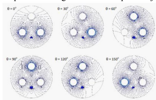
Gambar 9. Distribusi medan listrik dalam tangki GIS equilateral dengan keberadaan partikel k
