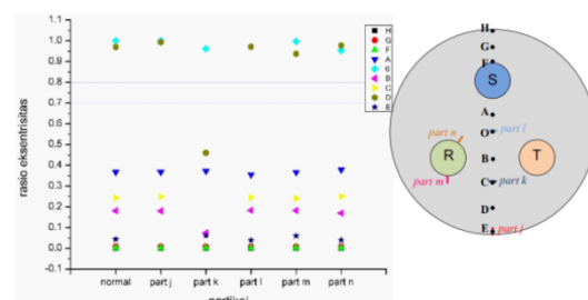
Gambar 21. Rasio eksentrisitas ( \eta ) di beberapa titik dengan variasi letak partikel
