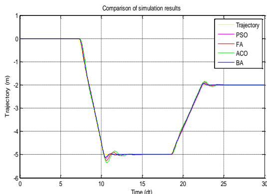
Gambar 5. Gambar lintasan masing-masing metode
