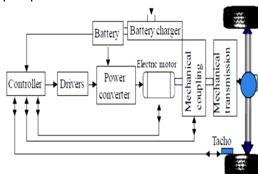
Gambar 2. Model elektrik kendaraan
